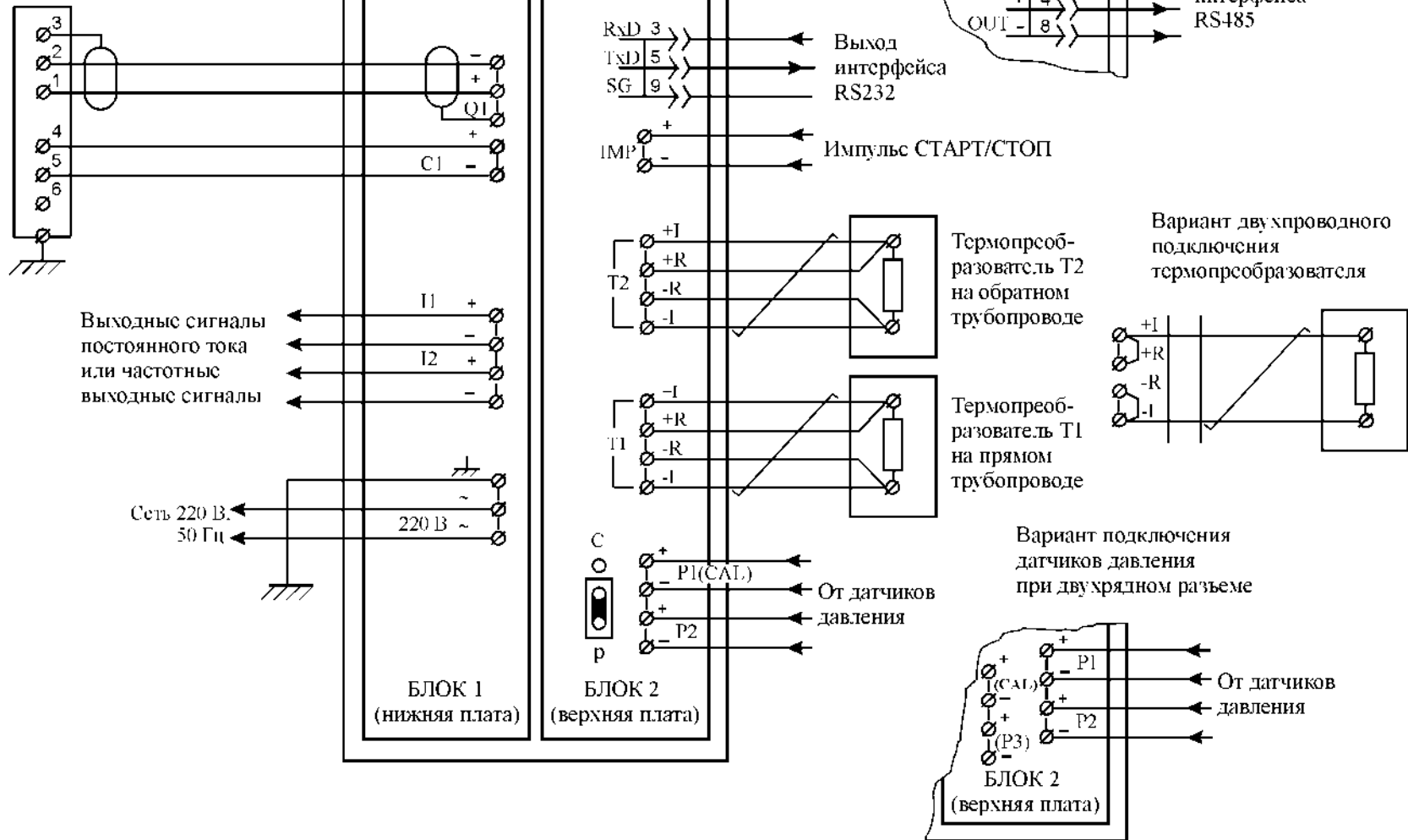
Рисунок 16 - Электрическая схема подключения теплосчетчика
