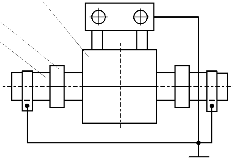
Рисунок 17 - Схема заземления первичных преобразователей
