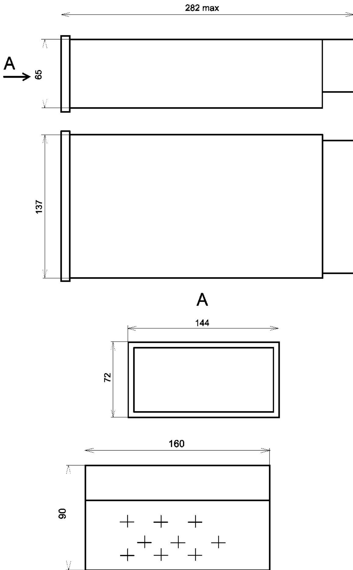
Рисунок 3 - габаритные и установочные размеры вычислительного блока щитового исполнения
